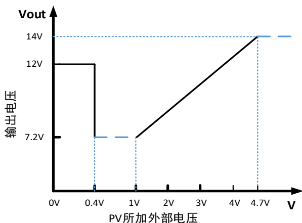
GW-1100W-48 主路输出 PV 调压曲线
