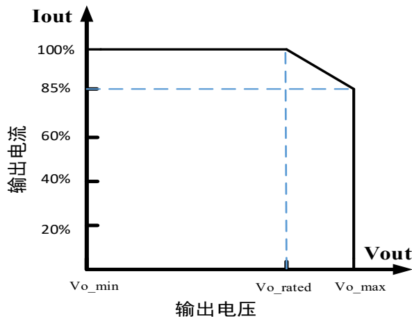
负载曲线
