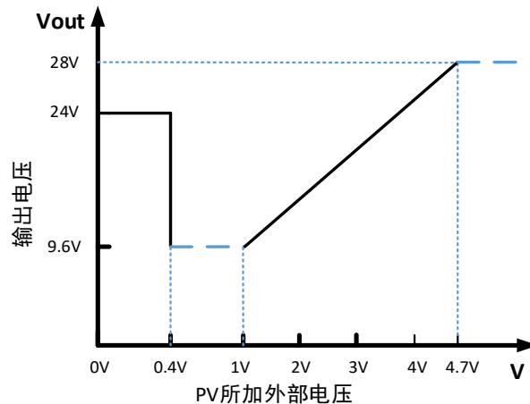
GW-1100W-24 主路输出 PV 调压曲线
