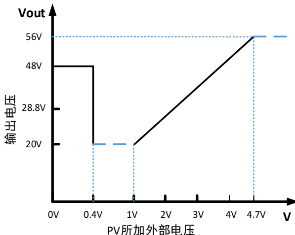
GW-1100W-48 主路输出 PV 调压曲线
