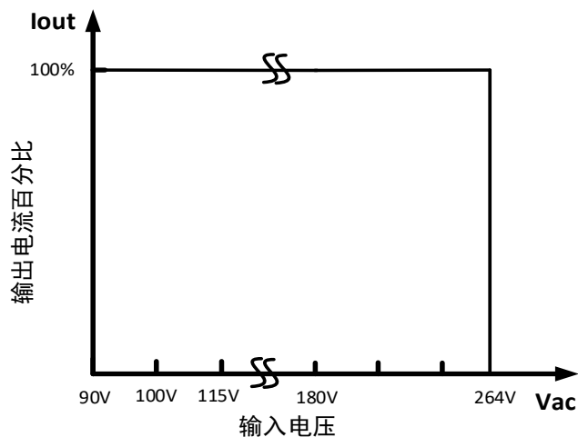
GW1100W-12V/24V/48V 输出降额曲线
