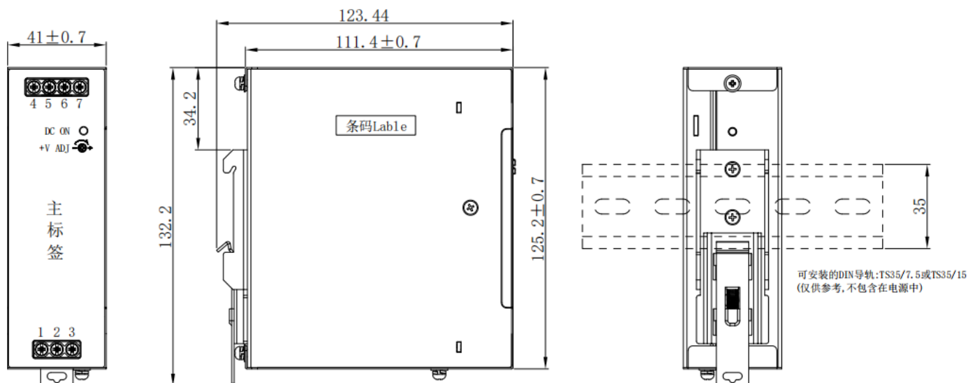
端子引脚分布 Terminal pin arrangement
