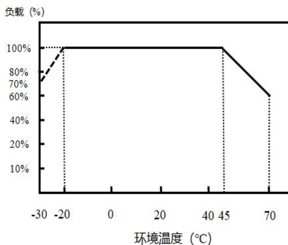
电源输出负载与最大支持环境温度关系
