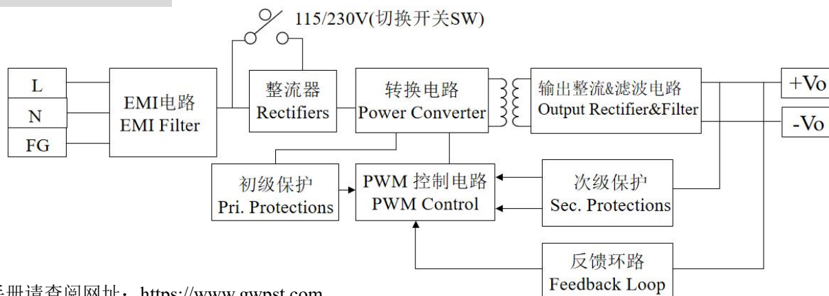
■ 方框图 Block Diagram
