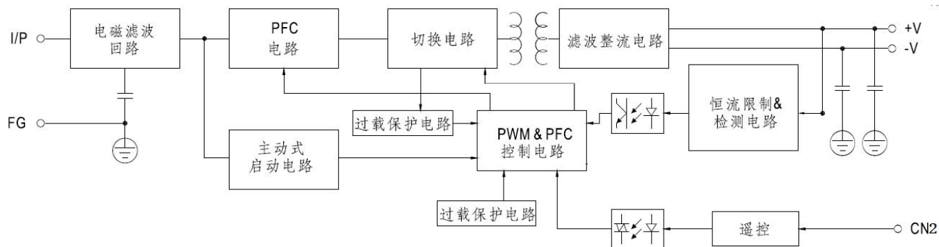
■ 方框图 Block Diagram
